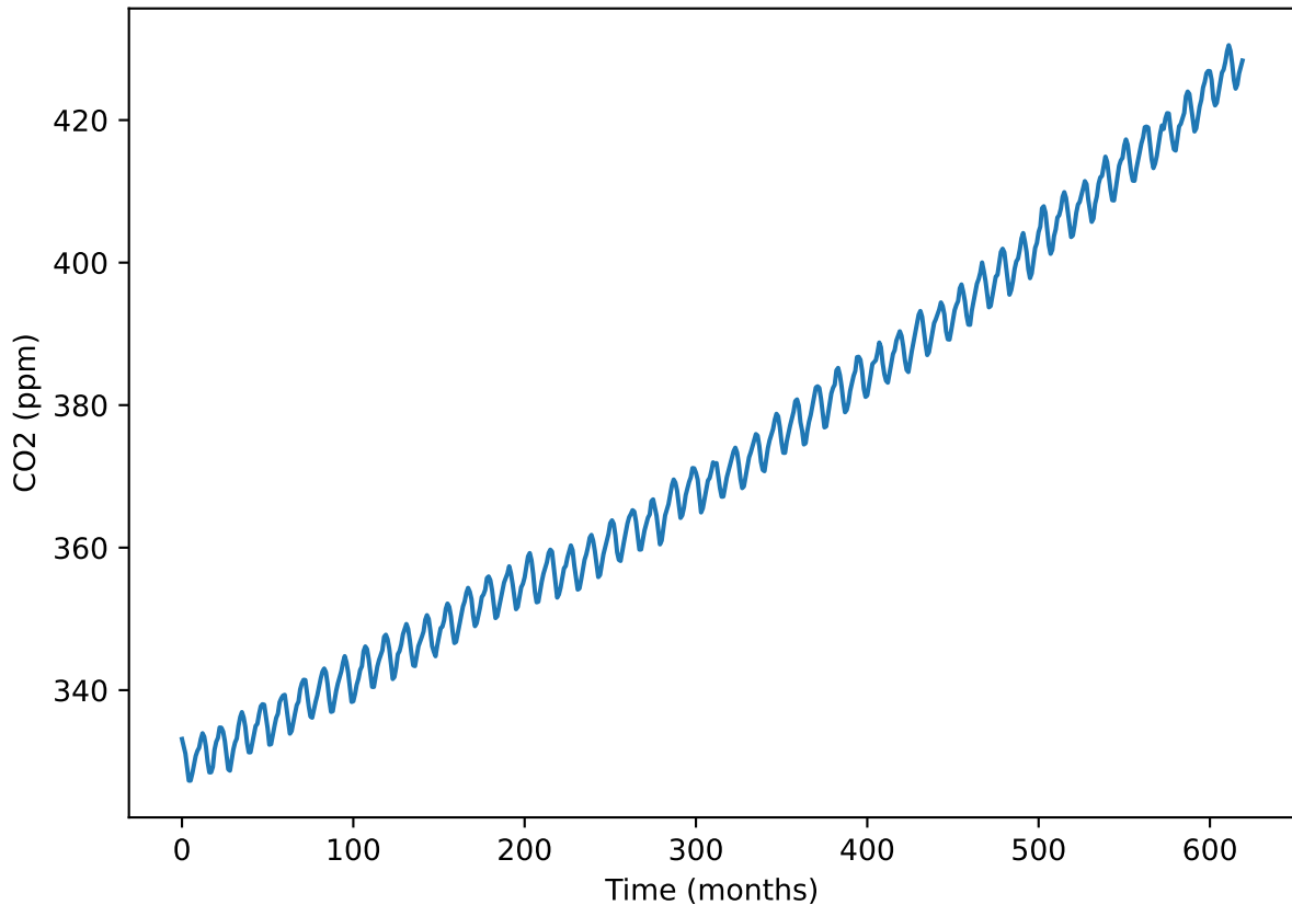
CO2 Monthly Mean
